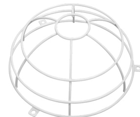
Grelha de proteção metálica BSK (Ø 200 x 90 mm) Número: 92199
