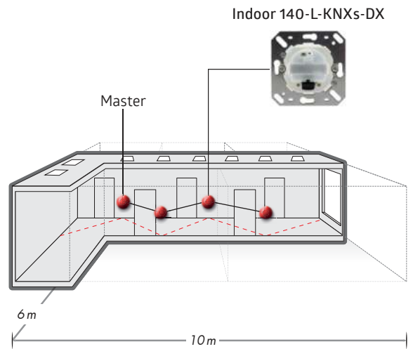
● Indoor 140-L-KNXs-DX - - - Erfassungsbereich sitzend
