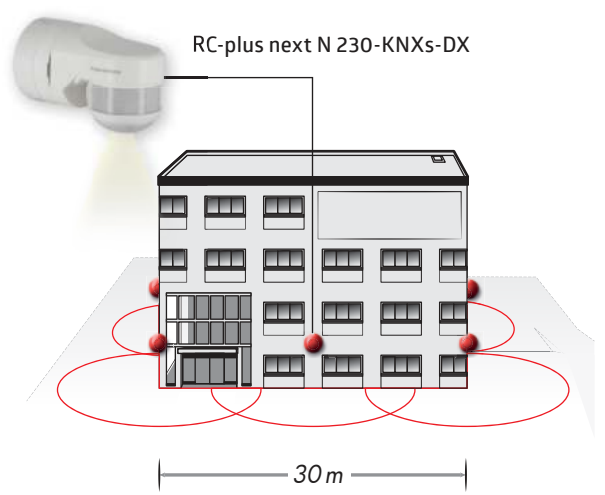
— Erfassungsbereich quer
