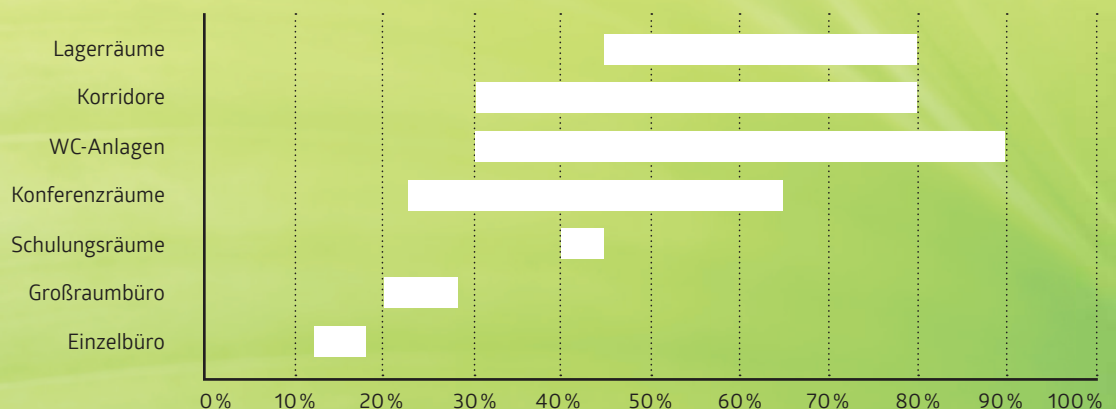
Möglichkeiten zur Energie- und Kostenreduktion mit Präsenzmeldern Energiesparpotential
