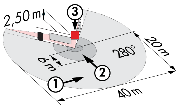
Reichweitendiagramm
