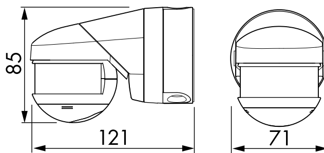
Bemaßung 97003
