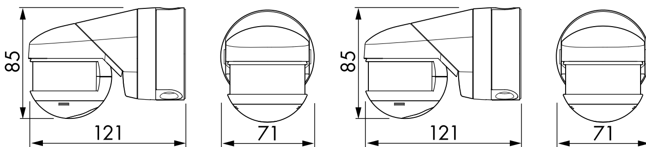
Bemaßung 97023
