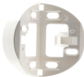
Zewnętrzna podstawka do montażu narożnego RC-plus next Nr art.: 97004
