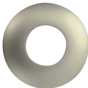
Fedőgyűrű PD9 Ø 45 mm Cikkszám: 92346
