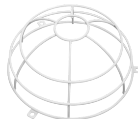
Védőrács BSK ( \varnothing 200 \times 90 mm) Art.No: 92199
