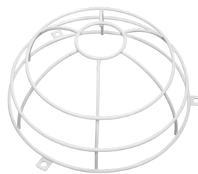
Panier de protection BSK ( \varnothing 200 \times 90 mm) Ref.: 92199
