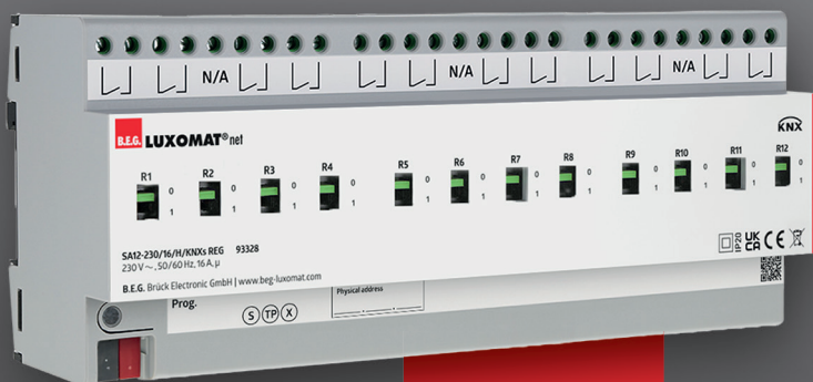
12-voudige schakelactor
