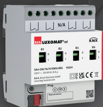
4-voudige schakelactor
