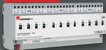
SA12-230/16/H/KNXs REG 12 schakeluitgangen Schakelactor
