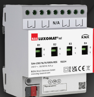
4-fach Schaltaktor
