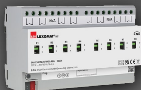
SA8-230/16/H/KNXs REG 8 spínacích výstupů Spínací aktor
