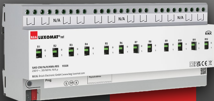
12-násobný spínací aktor
