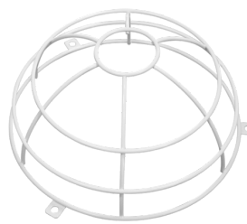
Ballschutzkorb BSK ( \varnothing 200 \times 90 mm) Art.No: 92199
