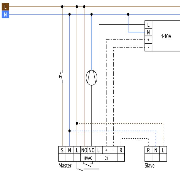
Wiring diagrams
